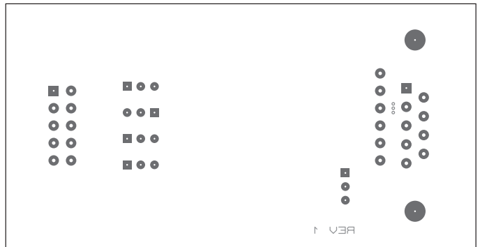
Layer 4. Bottom Layer
